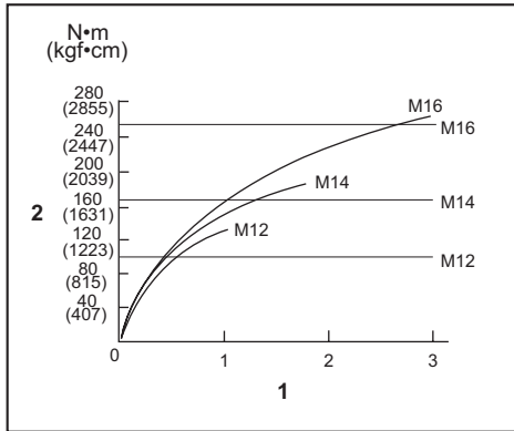
1. 紧固时间（秒） 2. 紧固转矩
