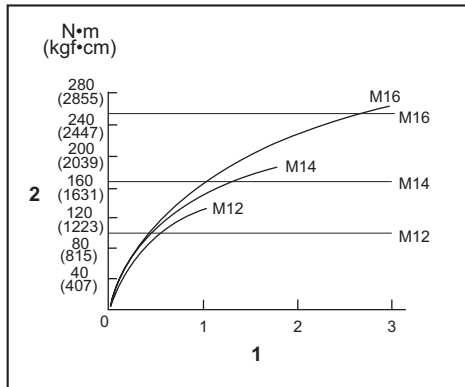
1. Waktu pengencangan (detik) 2. Torsi pengencangan
