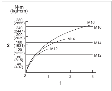
1. Thời gian vận xiết (giây) 2. Lực vận xiết
